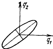
Рис. 85. Потенциальная энергия сильно связанных маятников
