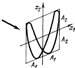
Рис. 19. Построение фигуры Лиссажу
