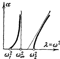
Рис. 86. Зависимость собственных частот от жесткости пружины
