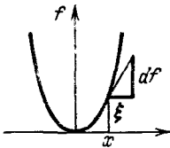
Рис. 140. Дифференциал функции
