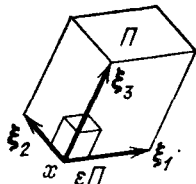
Рис. 155.* К определению дивергенции векторного поля
