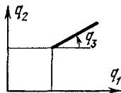
Рис. 59. Конфигурационное пространство отрезка на плоскости
