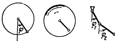
Рис. 58. Плоский, сферический и двойной маятники
