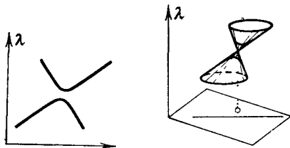
Рис. 243. Собственные частоты одно- и двухпараметрических семейств колебательных систем общего вида
