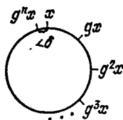
Рис. 52. Всюду плотное множество на окружности
