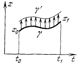
Рис. 41. Вариации кривой
