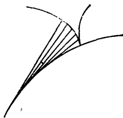
Рис. 252. Особенность звольвенты гладкой кривой
