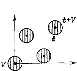
Рис. 213. К задаче 5
