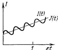
Рис. 224. Эволюция и осцилляции
