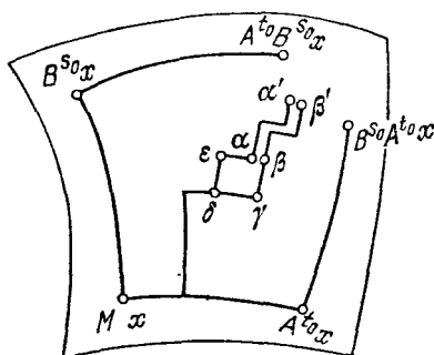
Рис. 171. Криволинейный четырехугольник \alpha\beta\gamma\delta\epsilon\alpha'
