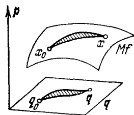
Рис. 219. Независимость интеграла \mathbf{p} d\mathbf{q} на M_f от пути
