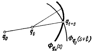
Рис. 194. Доказательство теоремы Гюйгенса
