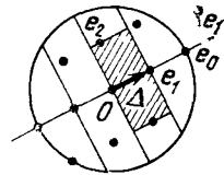
Рис. 215. К доказательству леммы о дискретных подгруппах
