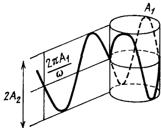
Рис. 19. Построение фигуры Лиссажу
