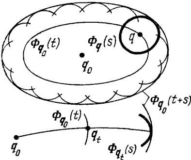
Рис. 193. Огибающая волновых фронтов
