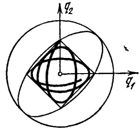
Рис. 82. Биения: траектория в конфигурационном пространстве
