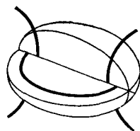
Рис. 249. Фокальный эллипс и фокальная гиперболы
