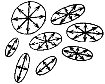
Рис. 192. Изотропная неоднородная среда
