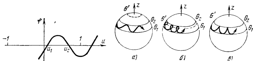
Рис. 127. График функции f(u)
