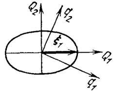
Рис. 78. Собственные колебания
