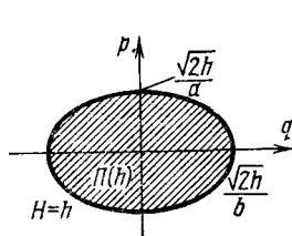
Рис. 217. Переменная действия для гармонического осциллятора
