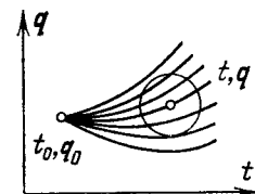
Рис. 198. Центральное поле экстремалей
