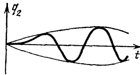
Рис. 83. Биения
