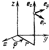
Рис. 145. К задаче 13
