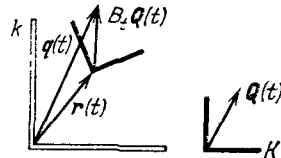
Рис. 104. Радиус-вектор точки относительно неподвижной ( q ) и подвижной ( Q ) системы координат
