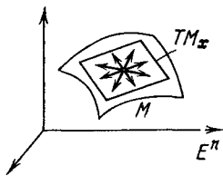
Рис. 62. Касательное пространство
