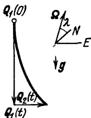
Рис. 109. Отклонение падающего камня силой Кориолиса
