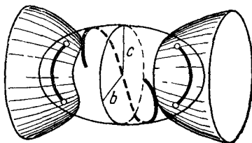
Рис. 208. Геодезические эллипсоида, касающиеся двухполостного гиперboloида
