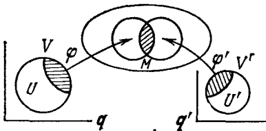
Рис. 56. Совместные карты
