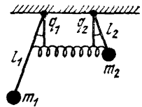
Рис. 84. Связанные маятники
