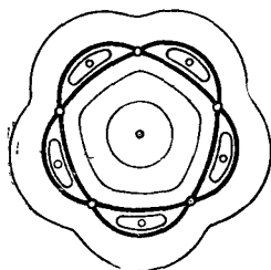
Рис. 241. Усредненный гамильтониан фазовых колебаний вблизи резонанса 5 : 1
