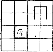
Рис. 160. Доказательство формулы Стокса для параллелепипеда
