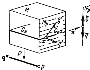
Рис. 238. Приведенное фазовое пространство
