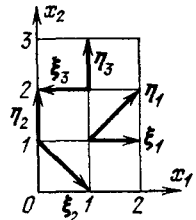
Рис. 143. К задаче 8
