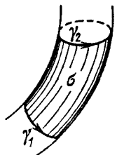
Рис. 180. Трубка ротора
