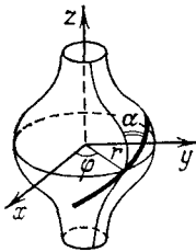
Рис. 66. Поверхность вращения
