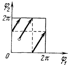
Рис. 221. Условно-периодическое движение
