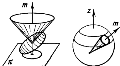
Рис. 131. Сравнение описаний движения волчка по Лагранжу и по Пуансо
