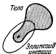
Рис. 116. Эллипсоид инерции
