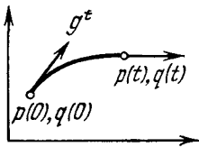
Рис. 47. Фазовый поток
