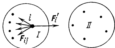
Рис. 39. Внутренние и внешние силы
