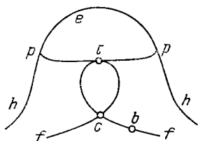
Рис. 259. Классификация точек на поверхности
