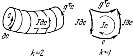
Рис. 167. След цепи при гомотопии
