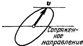
Рис. 196. Сопряженная гиперплоскость
