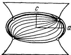
Рис. 207. Геодезические, выходящие из точек округления
