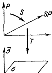
Рис. 209. К проверке невырожденности
