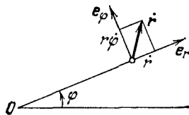
Рис. 29. Разложение вектора \dot{r} по базису e_r, e_\varphi
