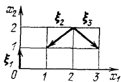
Рис. 142. К задаче 4
