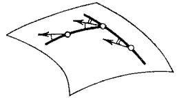
Рис. 230. Параллельное перенесение вдоль геодезической ломаной
