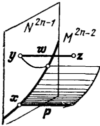
Рис. 179. Построение симплектических координат
