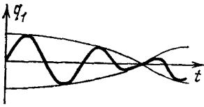
Рис. 83. Биения
