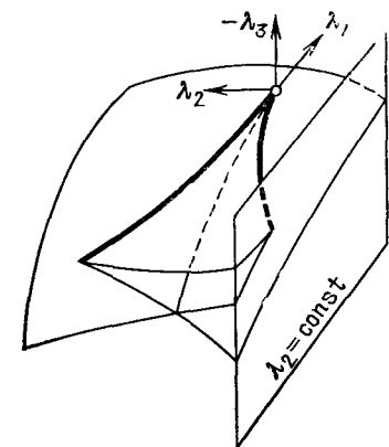
Рис. 247. Пуассонова структура пространства многочленов
