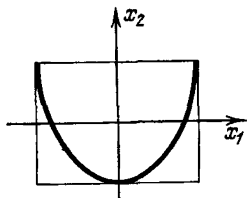
Рис. 22. Фигура Лиссажу с \omega = 2
