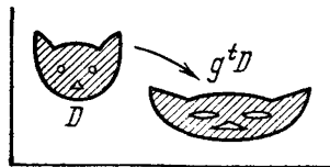
Рис. 48. Сохранение объема
