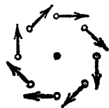
Рис. 27. Непотенциальное поле
