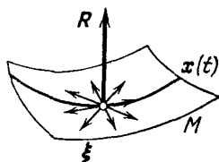
Рис. 71. Реакция связи
