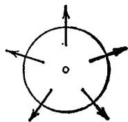
Рис. 163. Поле \mathbf{A}
