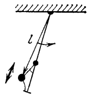
Рис. 94. Качели
