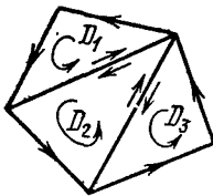
Рис. 161. Разбиение выпуклого многогранника на симплексы
