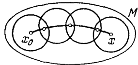
Рис. 212. К задаче 2
