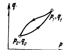
Рис. 185. Замкнутость формы p dq - PdQ
