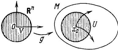
Рис. 211. К задаче 1
