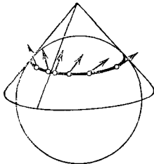
Рис. 231. Параллельное перенесение на сфере
