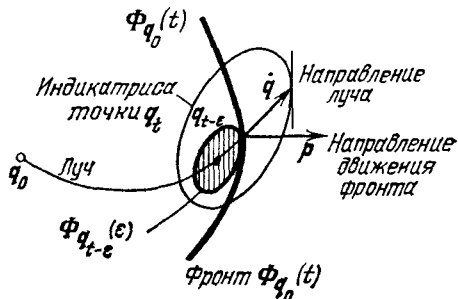
Рис. 197. Сопряженность направлений луча и фронта
