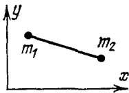
Рис. 65. Отрезок на плоскости
