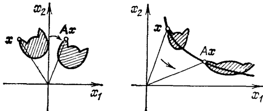
Рис. 96. Поворот и гиперболический поворот
