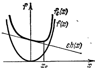
Рис. 132. Перемещение минимума при малом изменении функции
