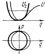
Рис. 76. Линеаризация
