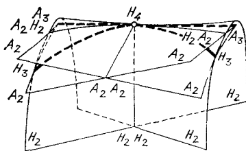
Рис. 268. Каустика группы H_4
