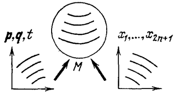
Рис. 184. Замена переменных в уравнениях Гамильтона
