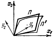
Рис. 159. Независимость внешней производной от системы координат
