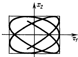
Рис. 21. Фигура Лиссажу с \omega \approx 1
