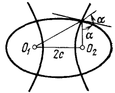
Рис. 204. Эллиптические координаты
