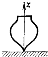
Рис. 129. Спящий волчок
