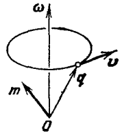
Рис. 114. Радиус-вектор, вектор скорости, угловая скорость и кинетический момент точки тела в пространстве
