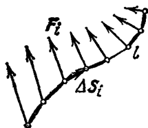
Рис. 26. Работа силового поля F на пути l
