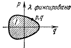
Рис. 228. Адиабатический инвариант, одномерной системы
