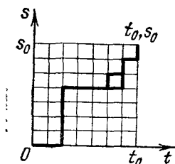
Рис. 170. К доказательству коммутативности потоков
