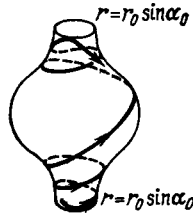
Рис. 67. Геодезические на поверхности вращения
