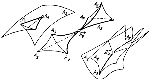
Рис. 246. Типичные особенности каустик в трехмерном пространстве
