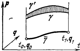
Рис. 187. Принцип наименьшего действия в фазовом пространстве
