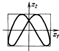
Рис. 23. Серия фигур Лиссажу с \omega = 2
