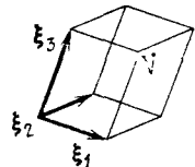
Рис. 138. Ориентированный объем — 3-форма
