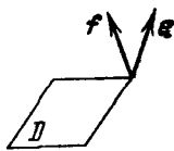
Рис. 174. Косоортогональное дополнение
