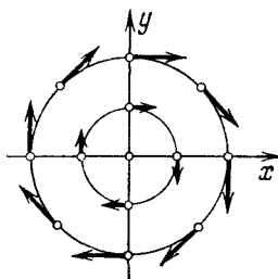
Рис. 9. Фазовая плоскость уравнения \ddot{x} = -x
