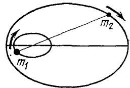
Рис. 40. Задача двух тел
