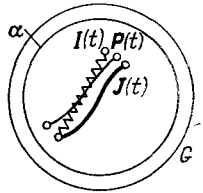
Рис. 226. Доказательство теоремы об усреднении
