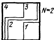
Рис. 172. Переход от одной пары сторон к другой
