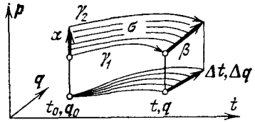
Рис. 200. Вычисление дифференциала функции действия.
