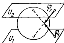
Рис. 57. Атлас сферы
