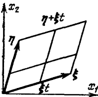
Рис. 158. К теореме о внешней производной
