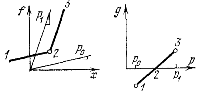
Рис. 44. Преобразование Лежандра переводит угол в отрезок
