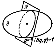
Рис. 91. Линейная связь
