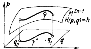
Рис. 189. Принцип Мопертюи
