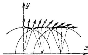
Рис. 232. Параллельное перенесение на плоскости Лобачевского
