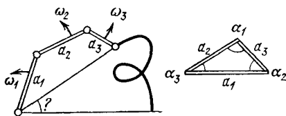
Рис. 223. К задаче о среднем движении перигелиев
