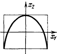
Рис. 23. Серия фигур Лиссажу с \omega = 2
