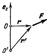
Рис. 37. Момент вектора F относительно оси
