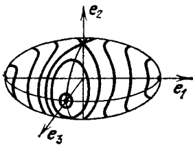
Рис. 121. Траектории уравнений Эйлера на поверхности уровня энергии
